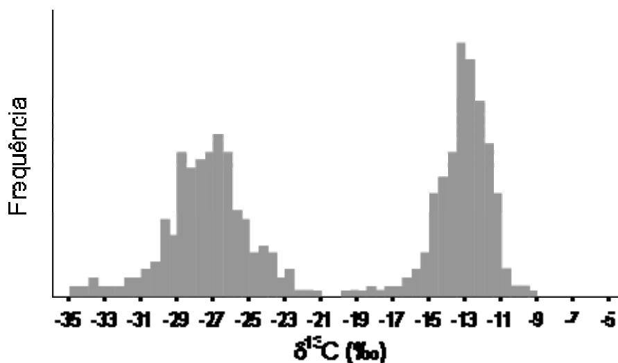
Figura 2. Histograma mostrando a distribuição de valores de \delta^{13}\text{C} em material vegetal, baseado em aproximadamente 1000 análises realizadas em diferentes laboratórios. (Modificada de O'leary 1988)
