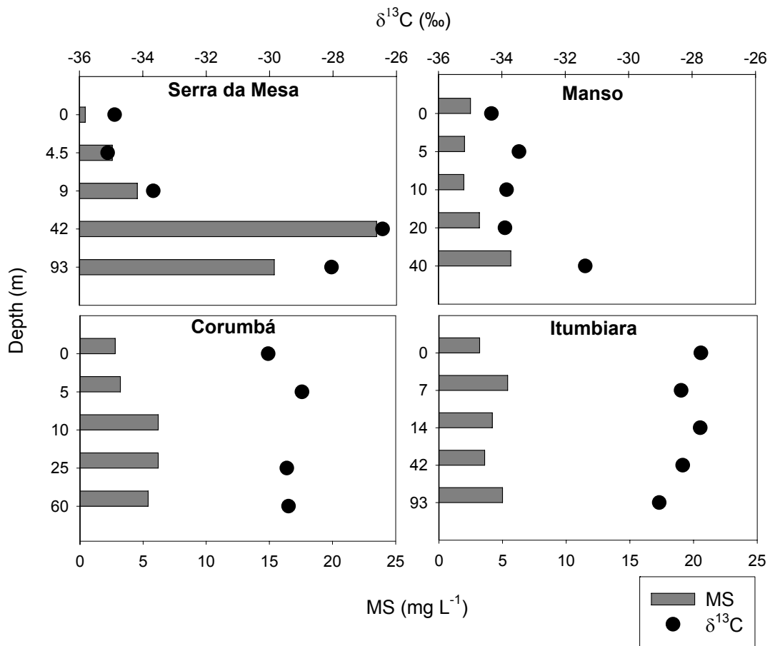
Figura 7. Concentração (mg L -1 ) e composição isotópica (δ 13 C) do material em suspensão nas amostragens em perfil de profundidade realizadas nos pontos próximos das barragens de cada reservatório.
