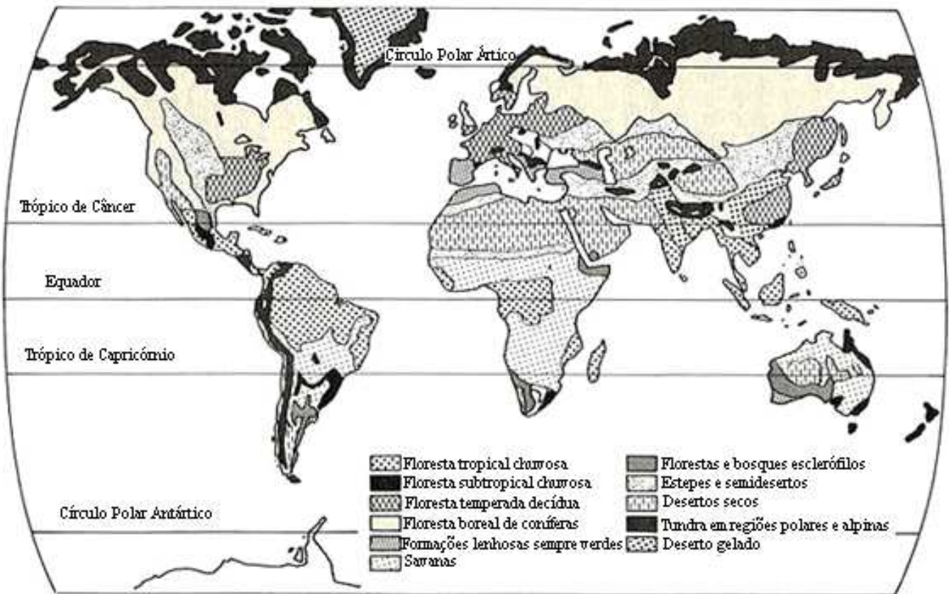
Mapa da distribuição das formações vegetacionais
