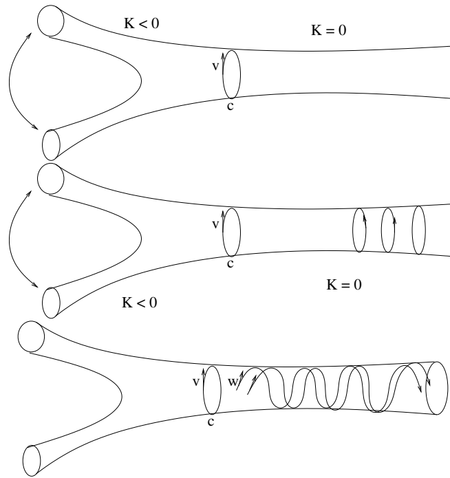
Figura 5.1: Exemplo 1
