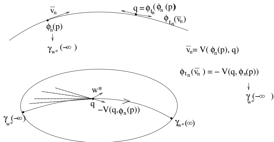
Figura 4.1: Lema 4.6
